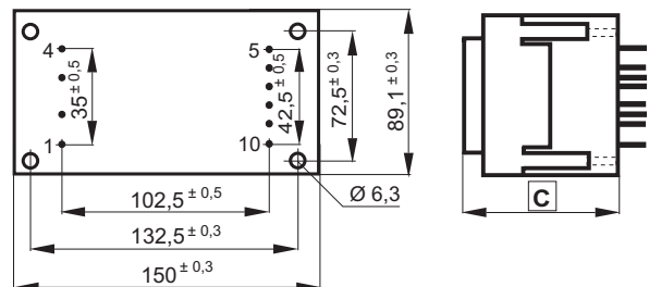
Ansicht auf Stiftseite - Pin view Abmessungen - Dimension in mm
